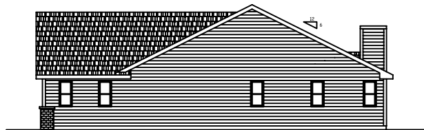
Right Elevation
